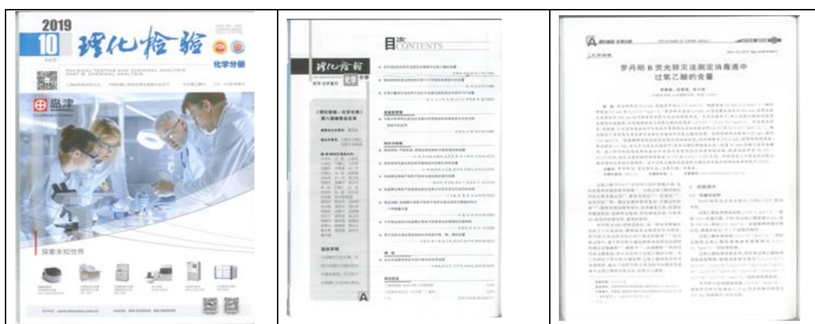
1. 罗丹明 B 荧光猝灭法测定消毒液中过氧乙酸的含量
